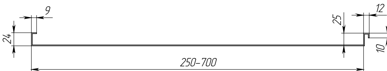
Фальцевая кровля
