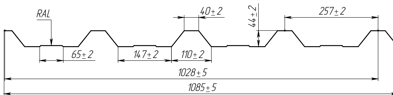
Профиль ПК-45
