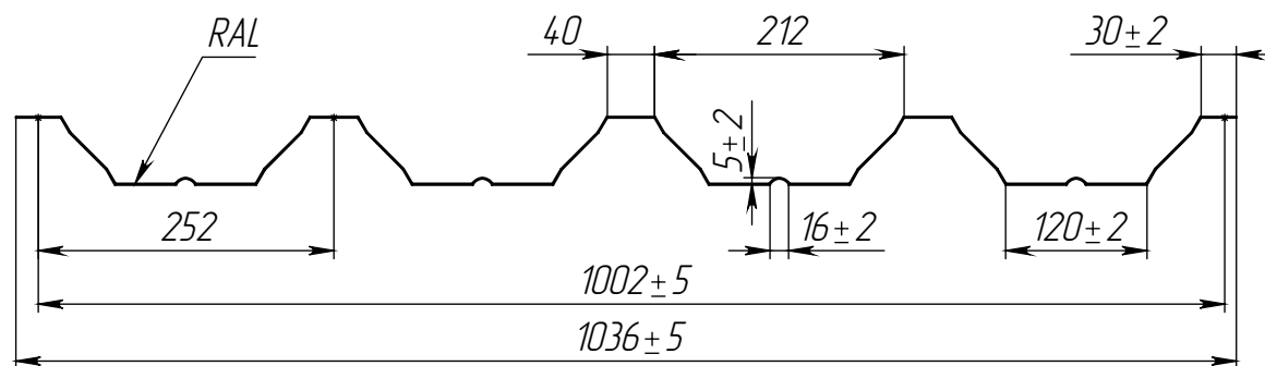
Профиль ПК-57
